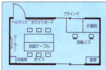
セットハウスSKH-40(4坪)例
