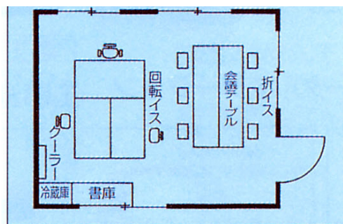
回送費用が軽減できる セットハウスSKH-53(5.3坪)例
